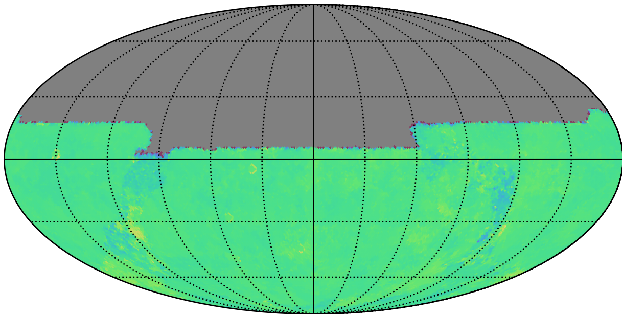
extra_ss_neo4_v3.4_10yrs u: Kuiper rotTelPos
