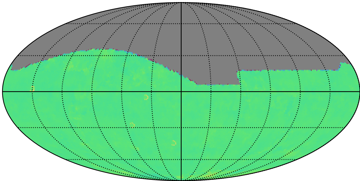
extra_ss_neo4_v3.4_10yrs r: Kuiper rotTelPos
