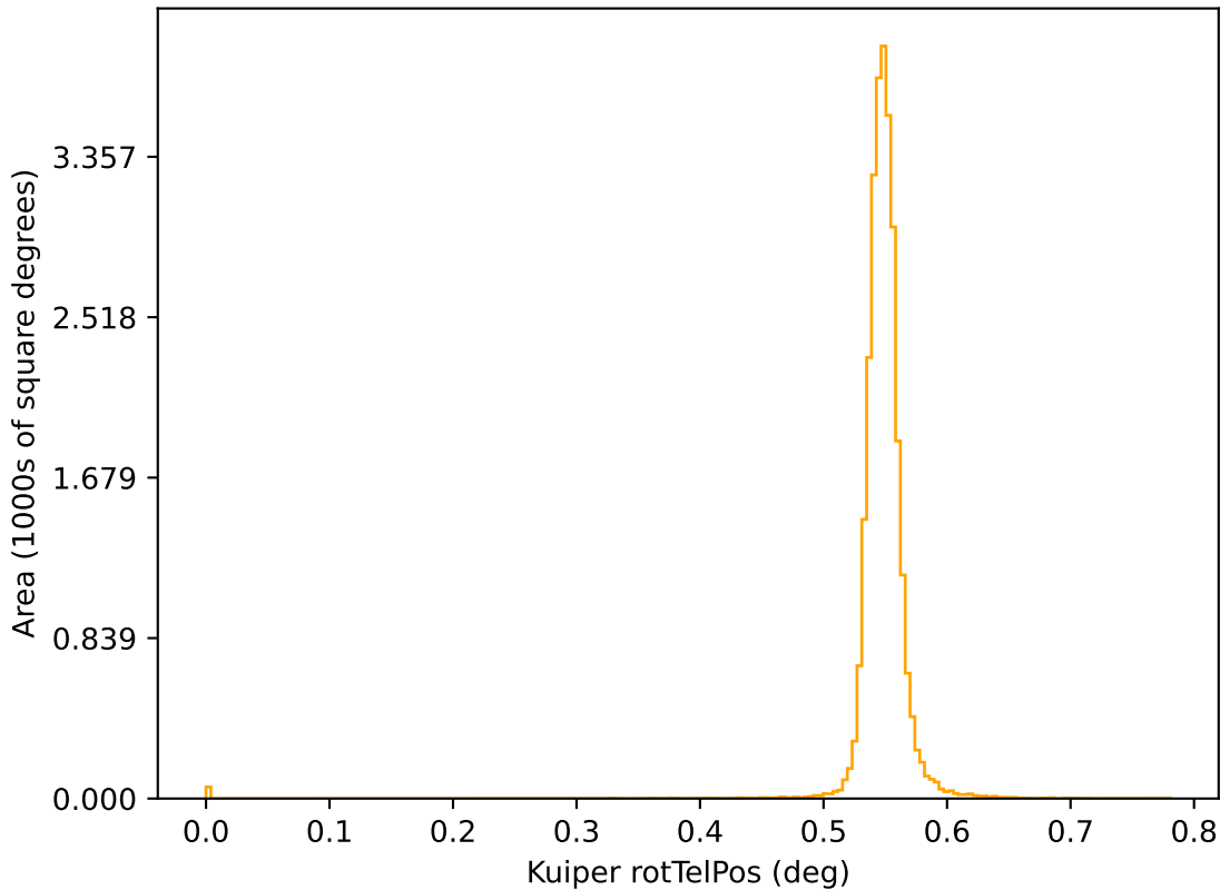
extra_ss_neo4_v3.4_10yrs r: Kuiper rotTelPos
