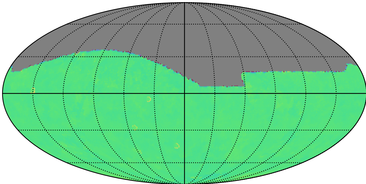
extra_ss_neo4_v3.4_10yrs i: Kuiper rotTelPos
