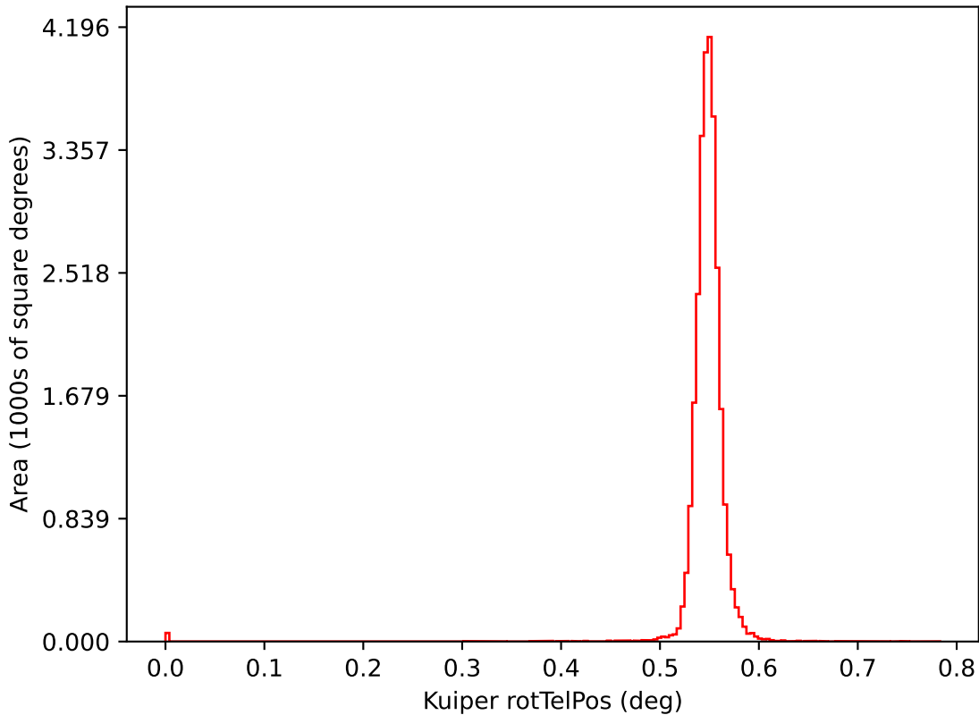
extra_ss_neo4_v3.4_10yrs i: Kuiper rotTelPos
