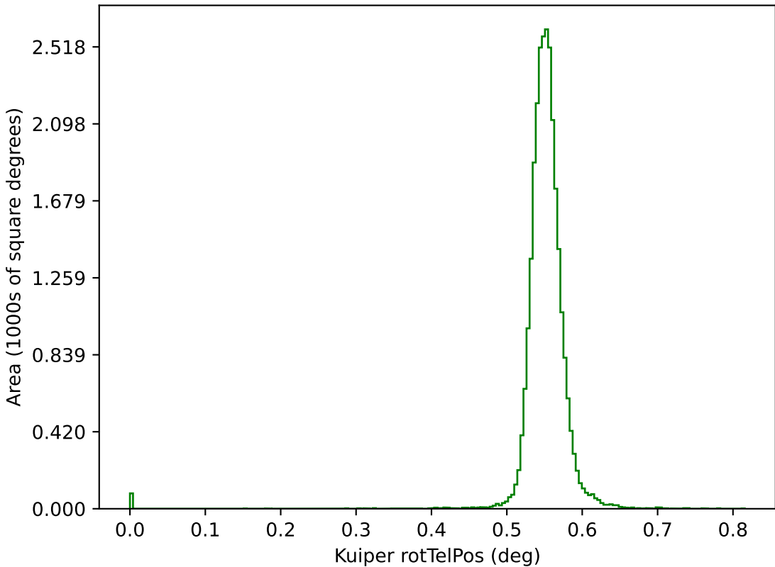
extra_ss_neo4_v3.4_10yrs g: Kuiper rotTelPos
