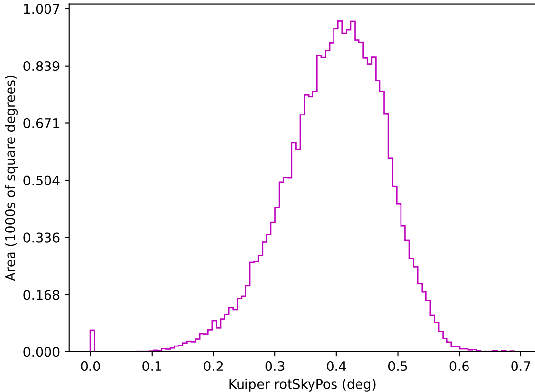
extra_ss_neo4_v3.4_10yrs z: Kuiper rotSkyPos
