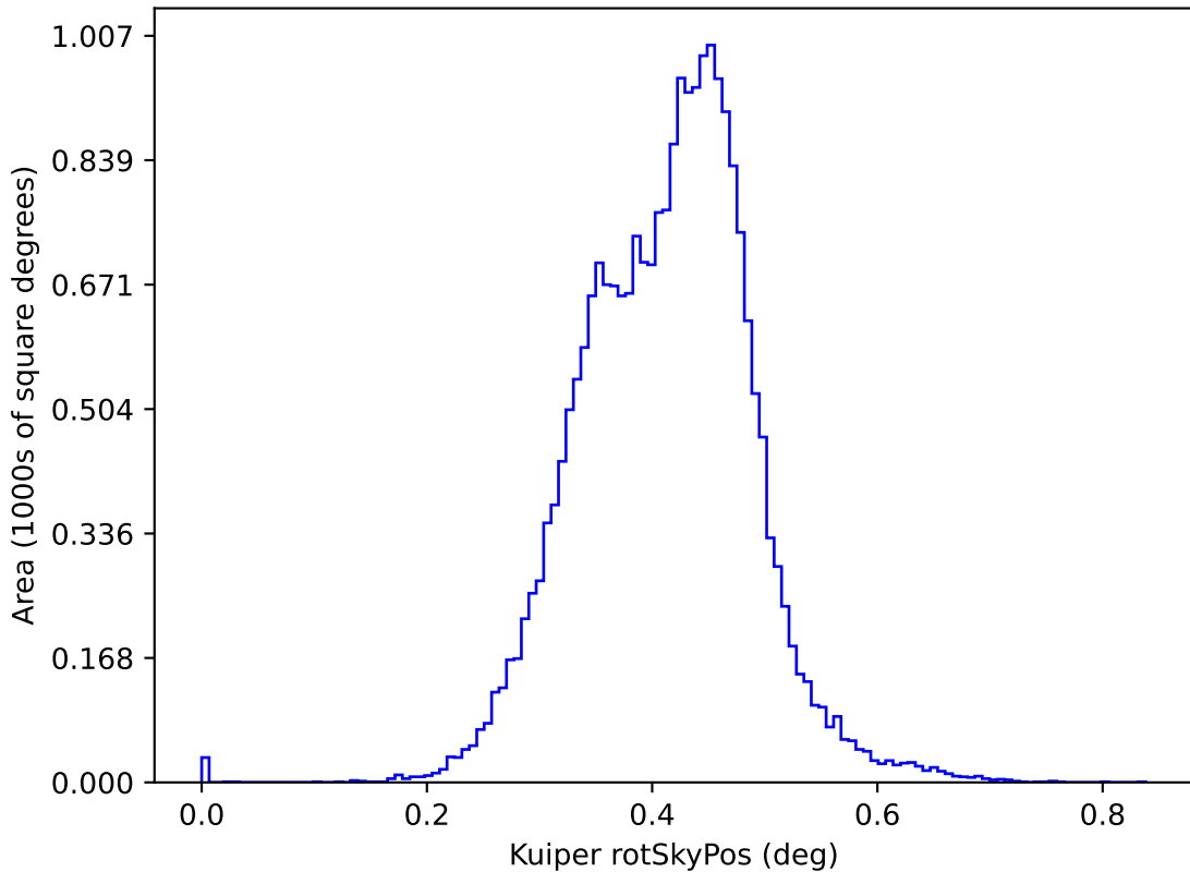
extra_ss_neo4_v3.4_10yrs y: Kuiper rotSkyPos
