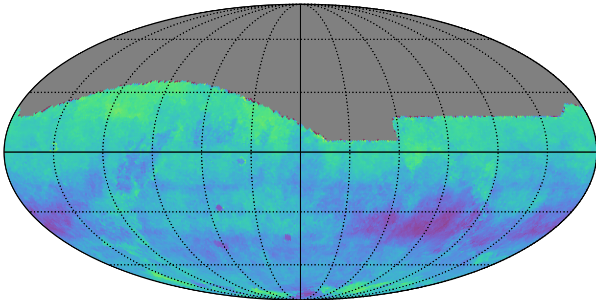
extra_ss_neo4_v3.4_10yrs r: Kuiper rotSkyPos
