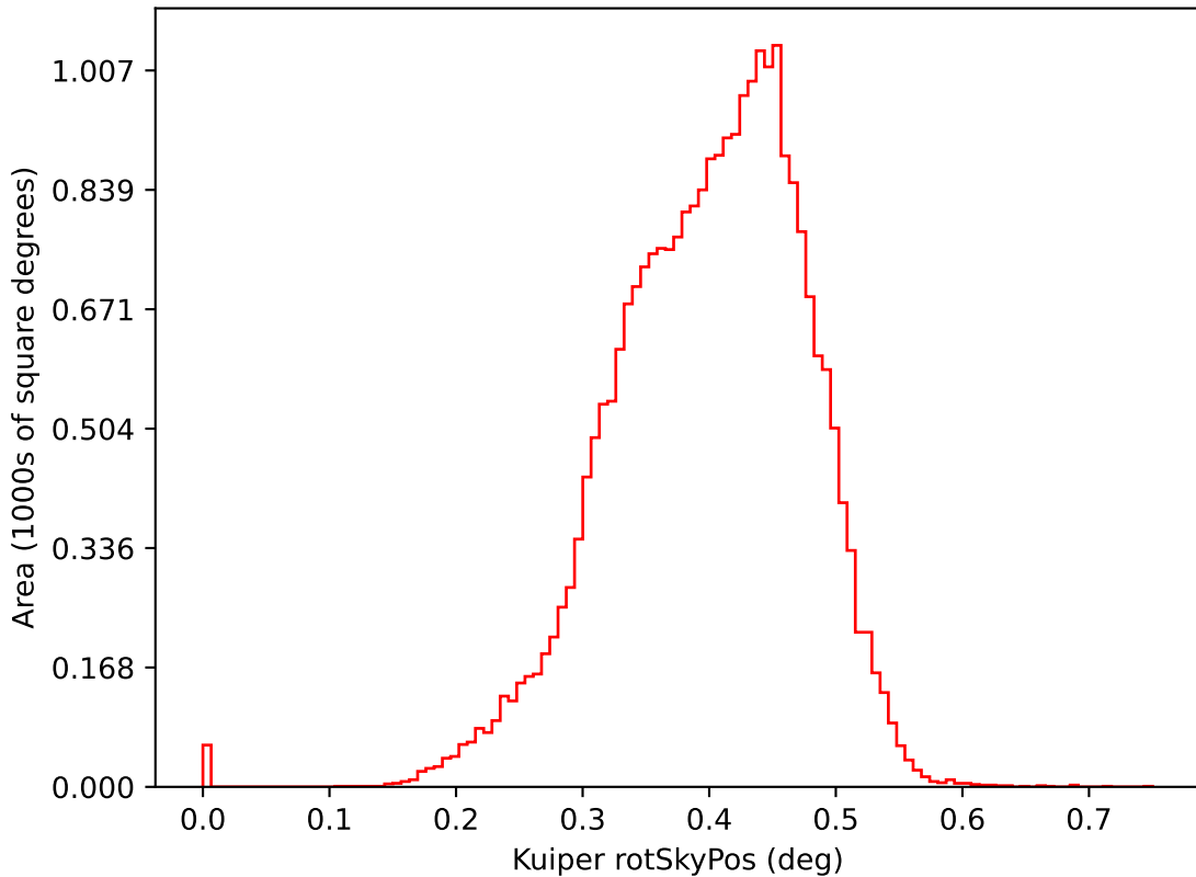
extra_ss_neo4_v3.4_10yrs i: Kuiper rotSkyPos
