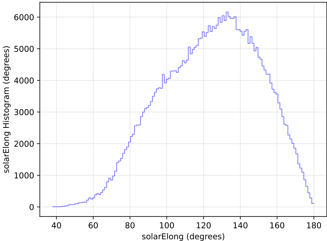
extra_ss_neo4_v3.4_10yrs WFD y band: solarElong Histogram
