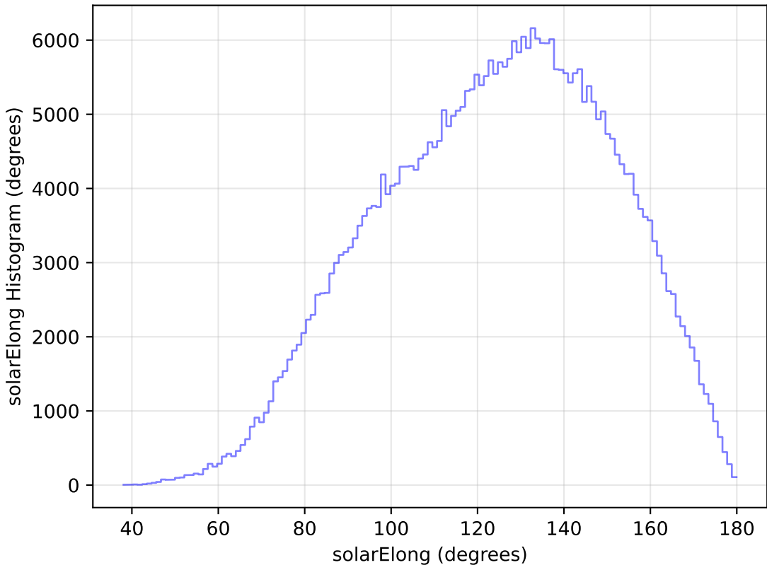
extra_ss_neo4_v3.4_10yrs All sky y band: solarElong Histogram
