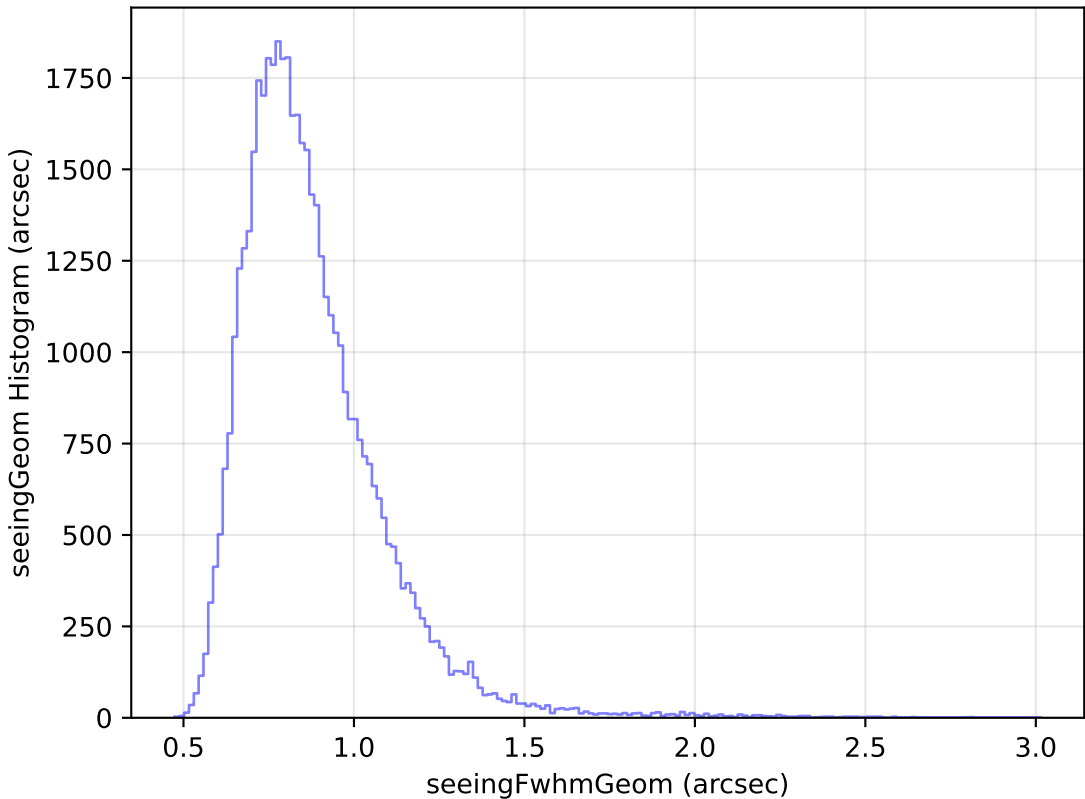
extra_ss_neo4_v3.4_10yrs Yr 1 y band: seeingGeom Histogram
