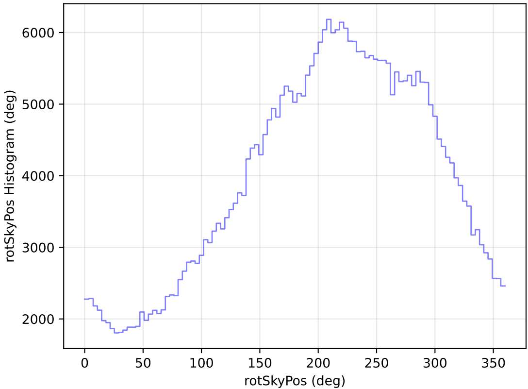
extra_ss_neo4_v3.4_10yrs WFD y band: rotSkyPos Histogram
