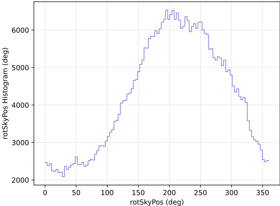
extra_ss_neo4_v3.4_10yrs All sky z band: rotSkyPos Histogram
