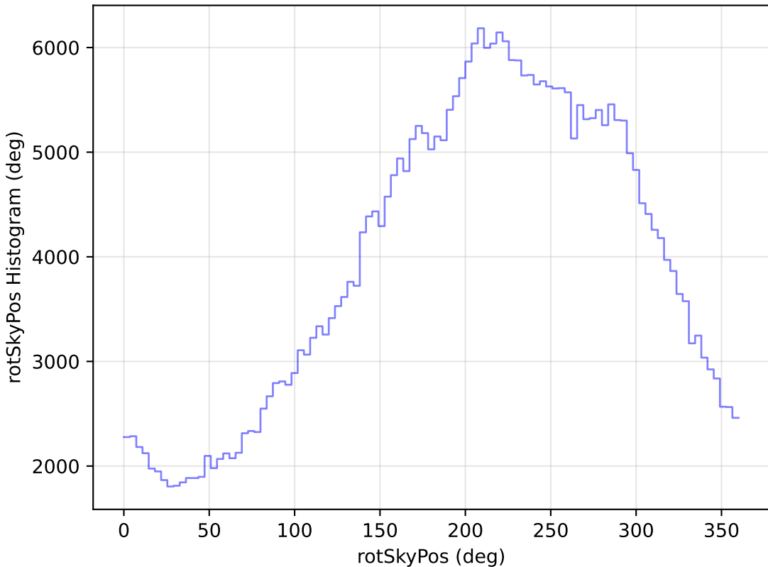
extra_ss_neo4_v3.4_10yrs All sky y band: rotSkyPos Histogram
