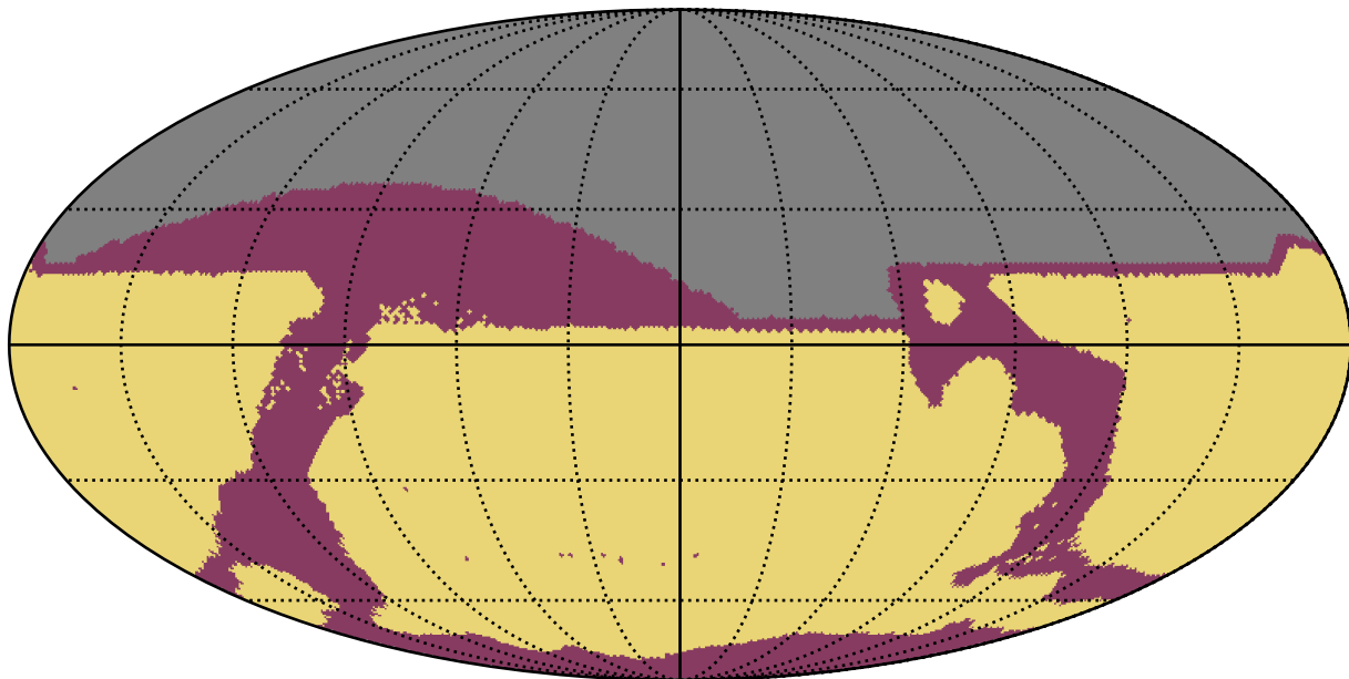
extra_ss_neo4_v3.4_10yrs All sky: RapidRevisits
