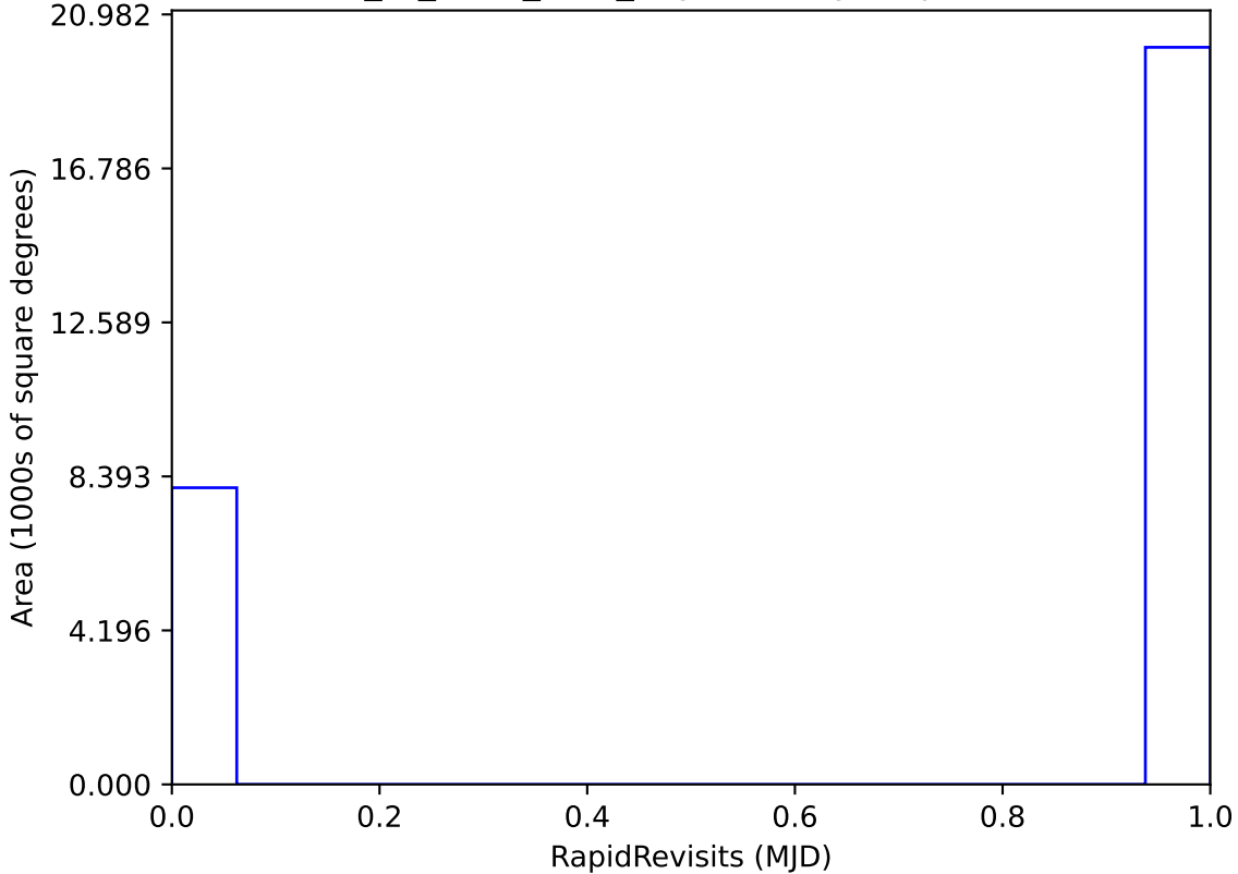
extra_ss_neo4_v3.4_10yrs All sky: RapidRevisits
