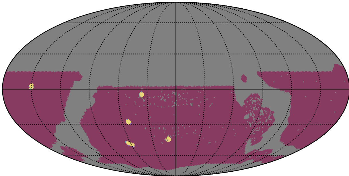
extra_ss_neo4_v3.4_10yrs WFD: NumberOfQuickRevisits
