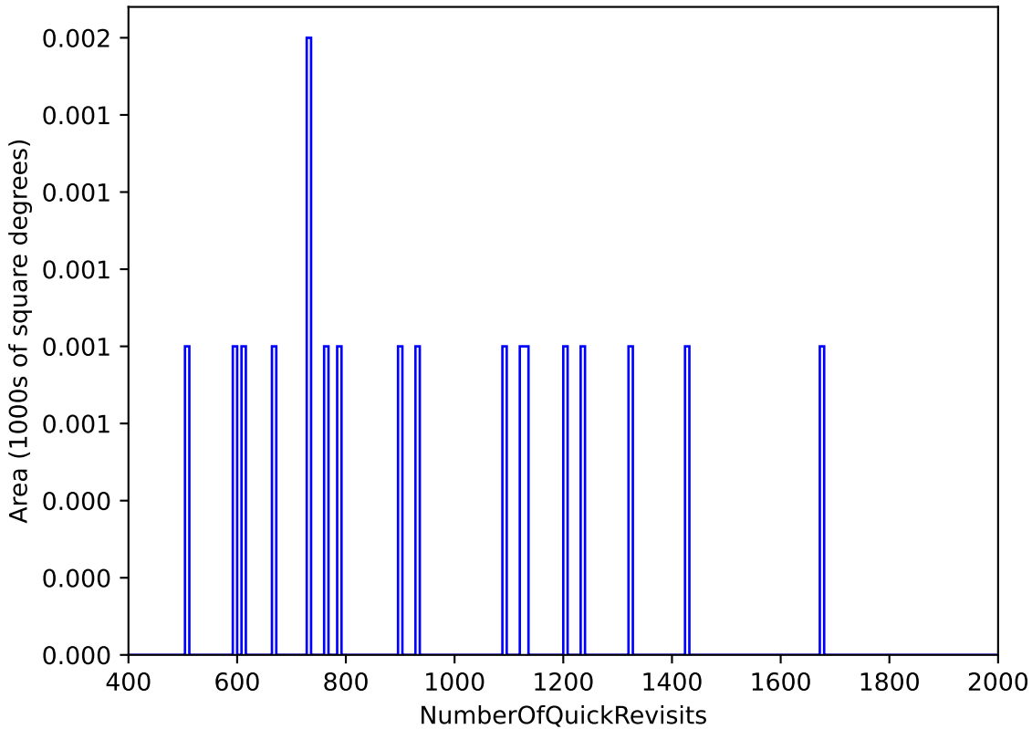
extra_ss_neo4_v3.4_10yrs WFD: NumberOfQuickRevisits
