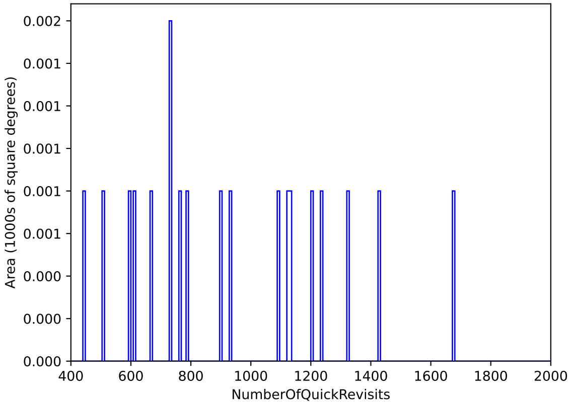
extra_ss_neo4_v3.4_10yrs All sky: NumberOfQuickRevisits
