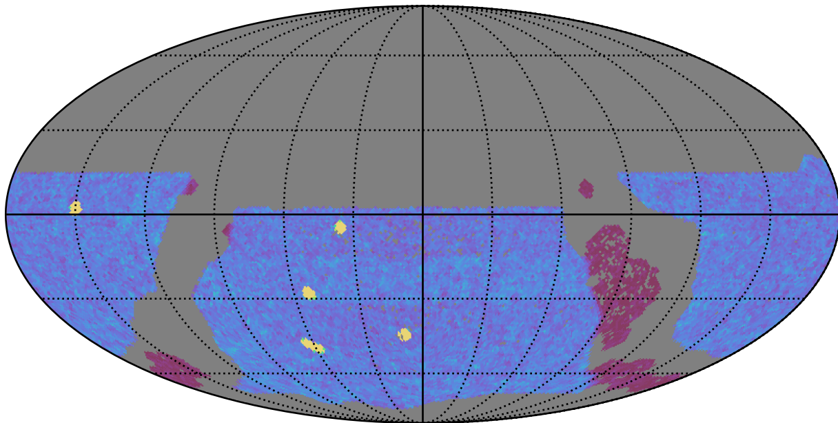
extra_ss_neo4_v3.4_10yrs WFD y band: NVisits
