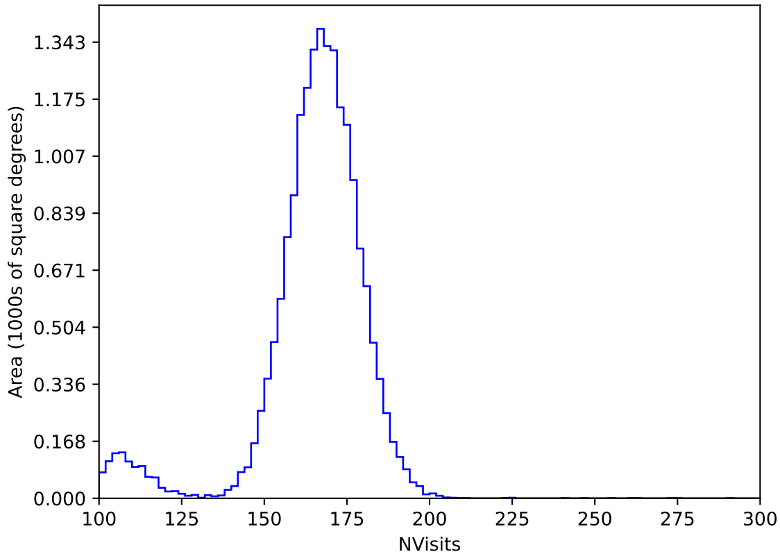
extra_ss_neo4_v3.4_10yrs WFD y band: NVisits
