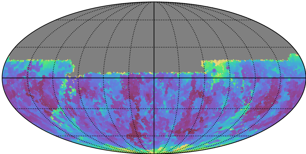
extra_ss_neo4_v3.4_10yrs Yr 1 y band: Min seeingEff
