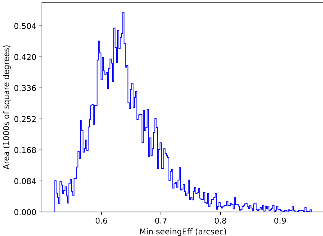
extra_ss_neo4_v3.4_10yrs All sky y band: Min seeingEff
