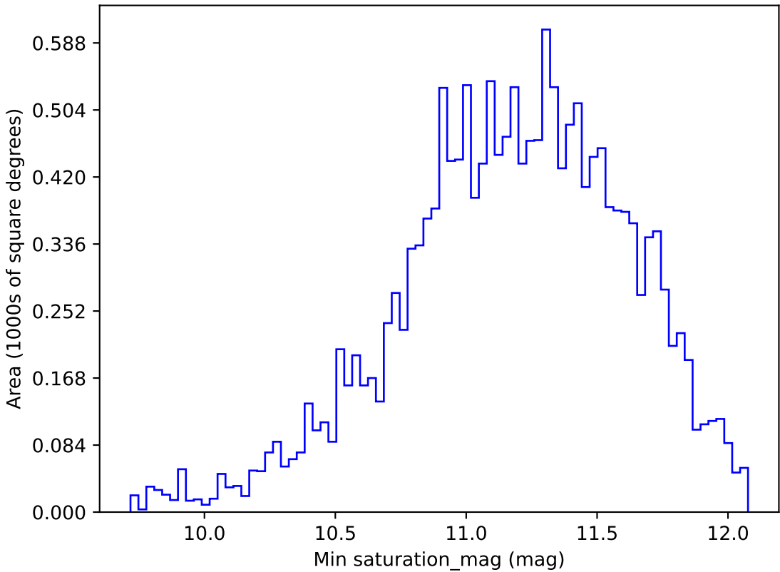
extra_ss_neo4_v3.4_10yrs WFD y band: Min saturation_mag
