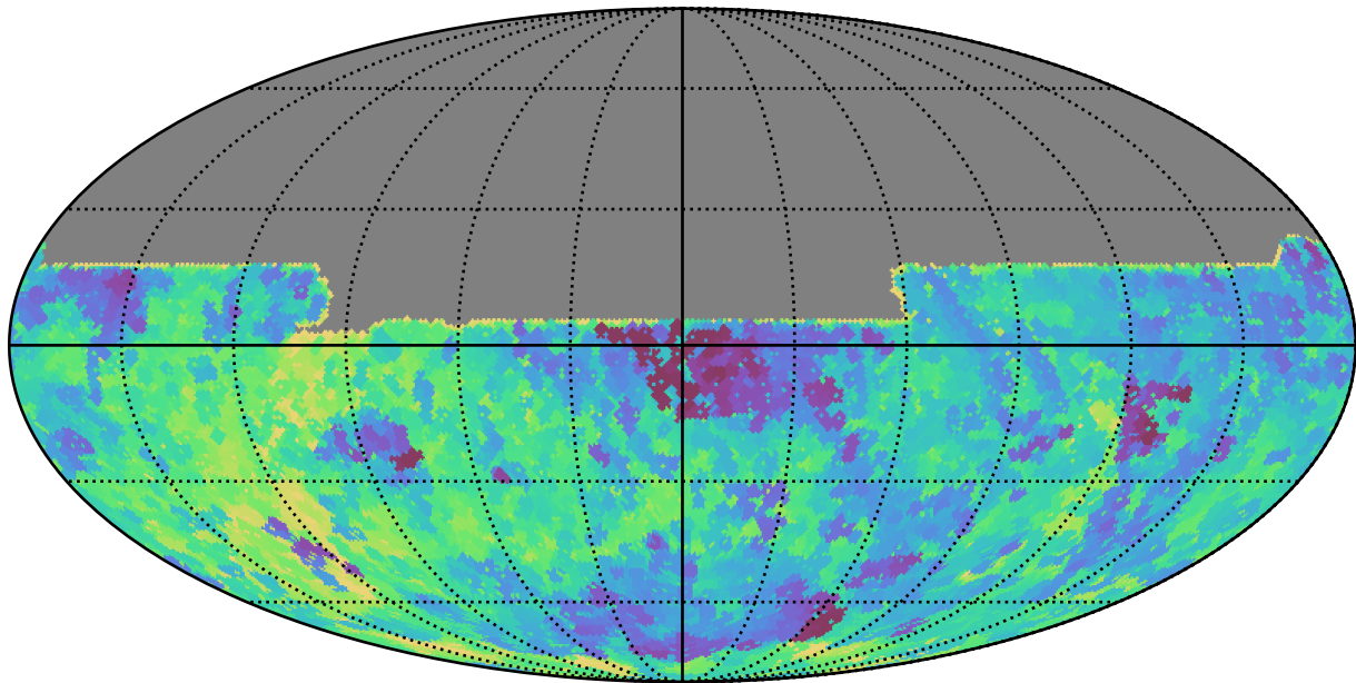
extra_ss_neo4_v3.4_10yrs All sky y band: Min saturation_mag
