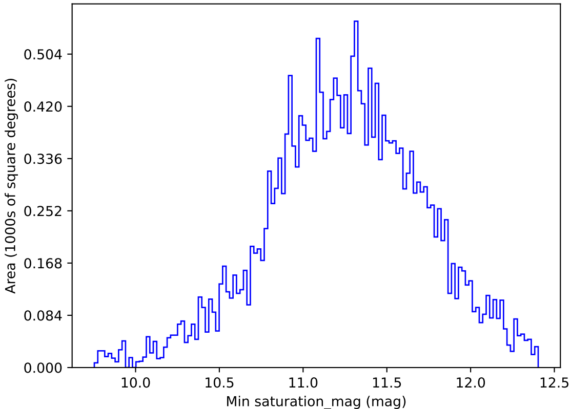
extra_ss_neo4_v3.4_10yrs All sky y band: Min saturation_mag
