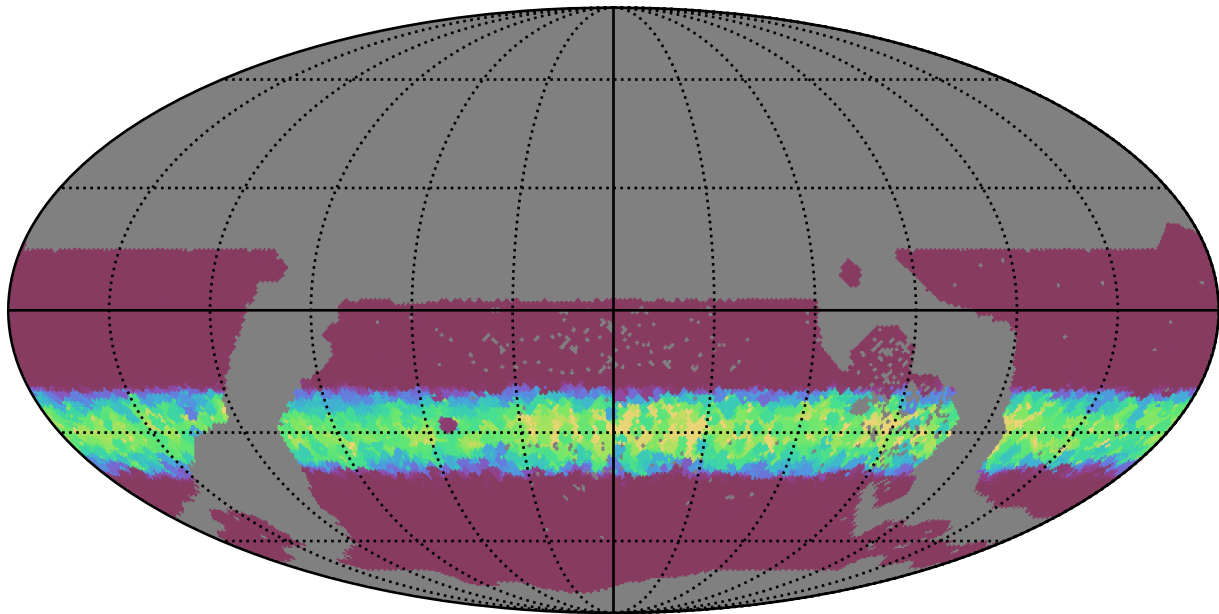
extra_ss_neo4_v3.4_10yrs WFD z band: Min normairmass
