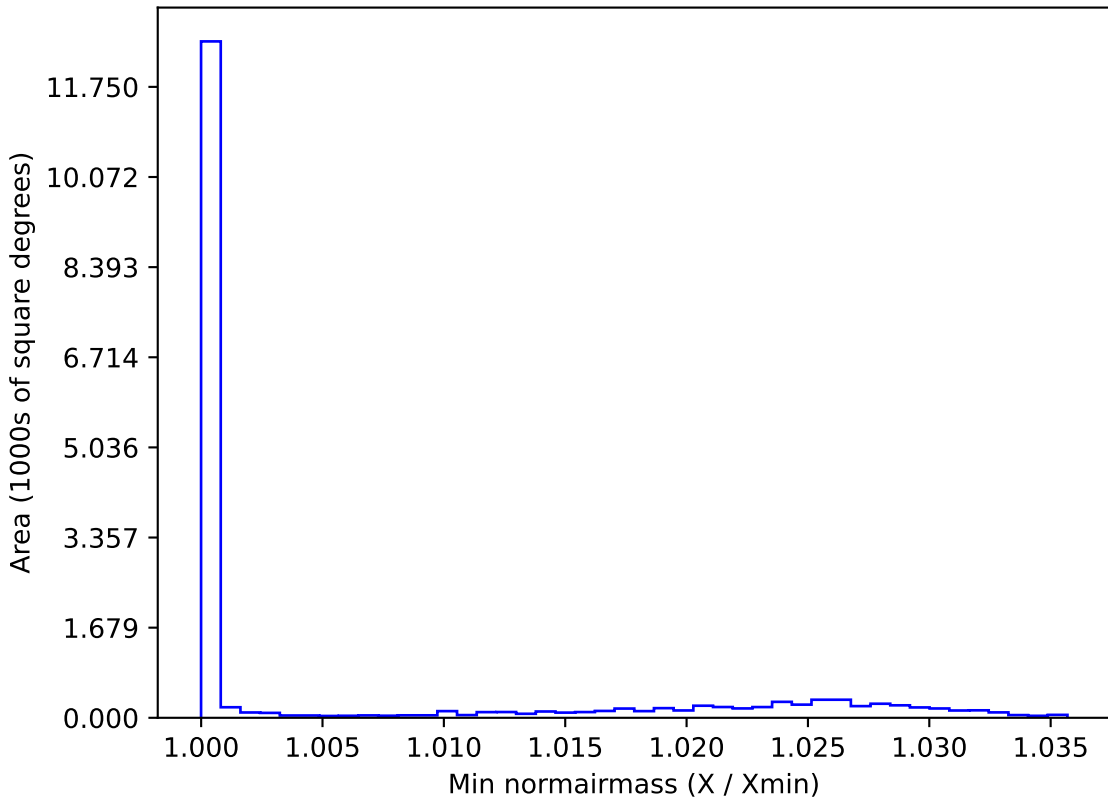
extra_ss_neo4_v3.4_10yrs WFD z band: Min normairmass
