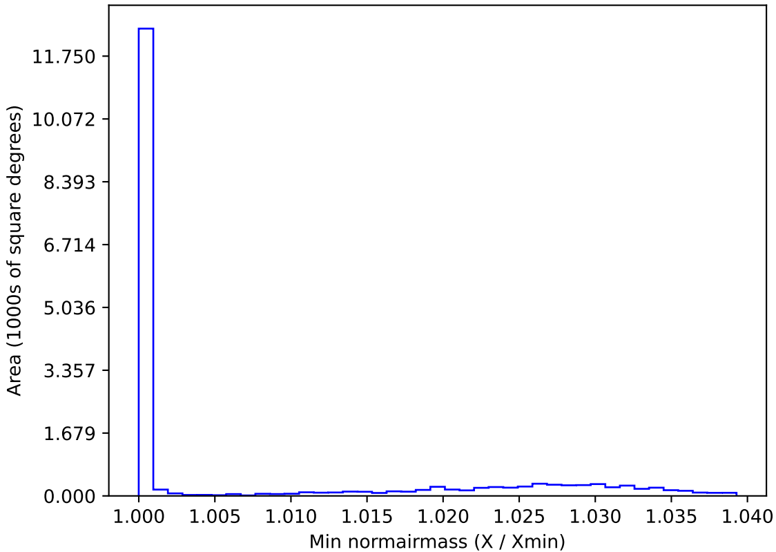
extra_ss_neo4_v3.4_10yrs WFD y band: Min normairmass
