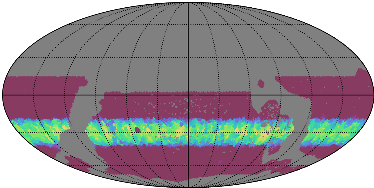
extra_ss_neo4_v3.4_10yrs WFD g band: Min normairmass
