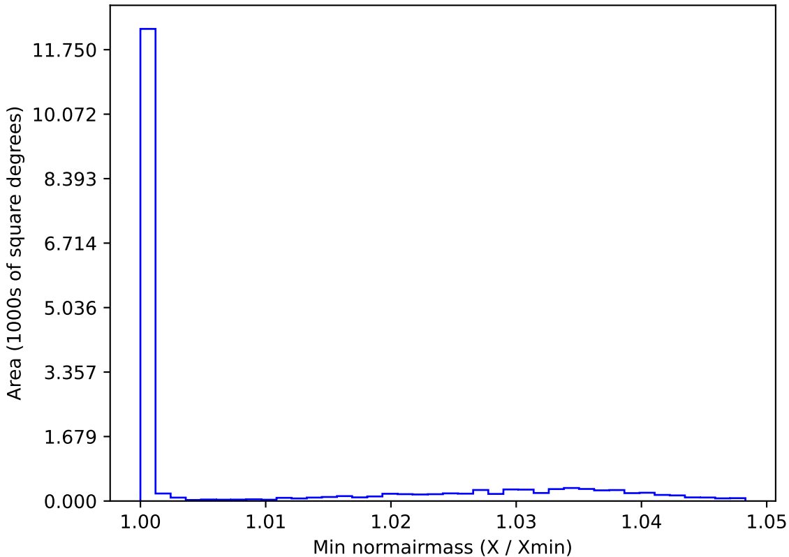
extra_ss_neo4_v3.4_10yrs WFD g band: Min normairmass
