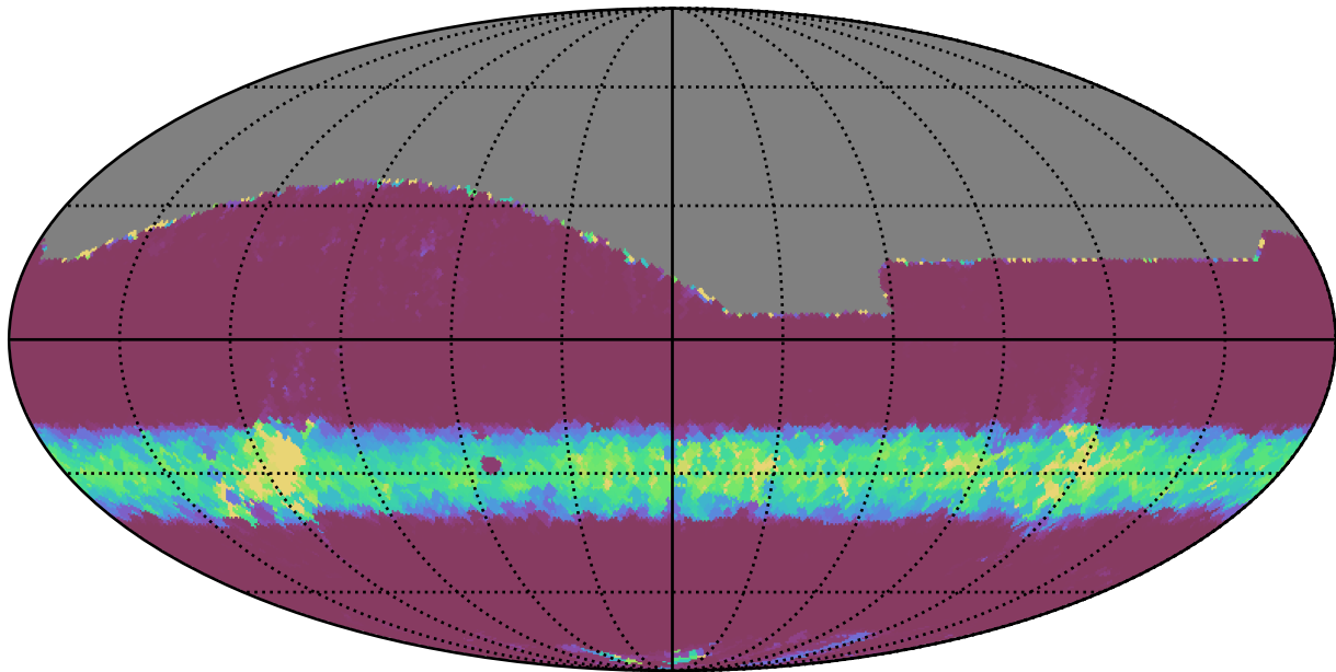
extra_ss_neo4_v3.4_10yrs All sky z band: Min normairmass
