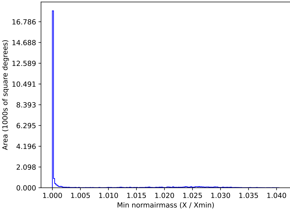
extra_ss_neo4_v3.4_10yrs All sky z band: Min normairmass
