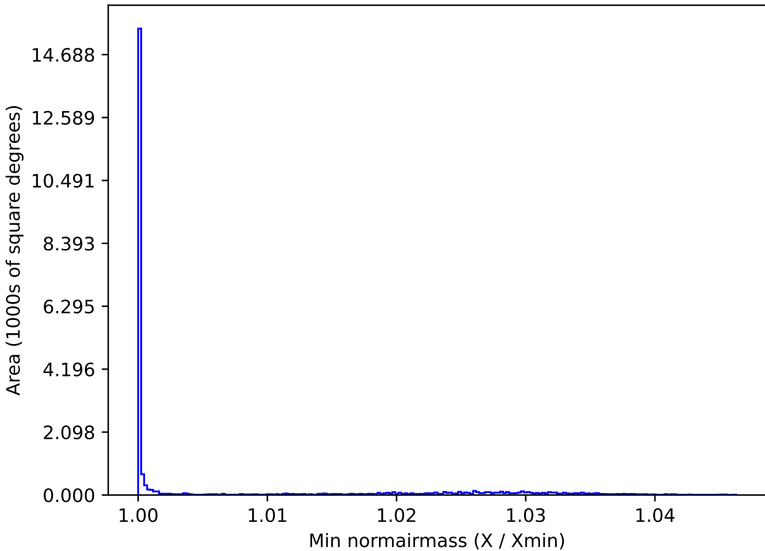
extra_ss_neo4_v3.4_10yrs All sky y band: Min normairmass
