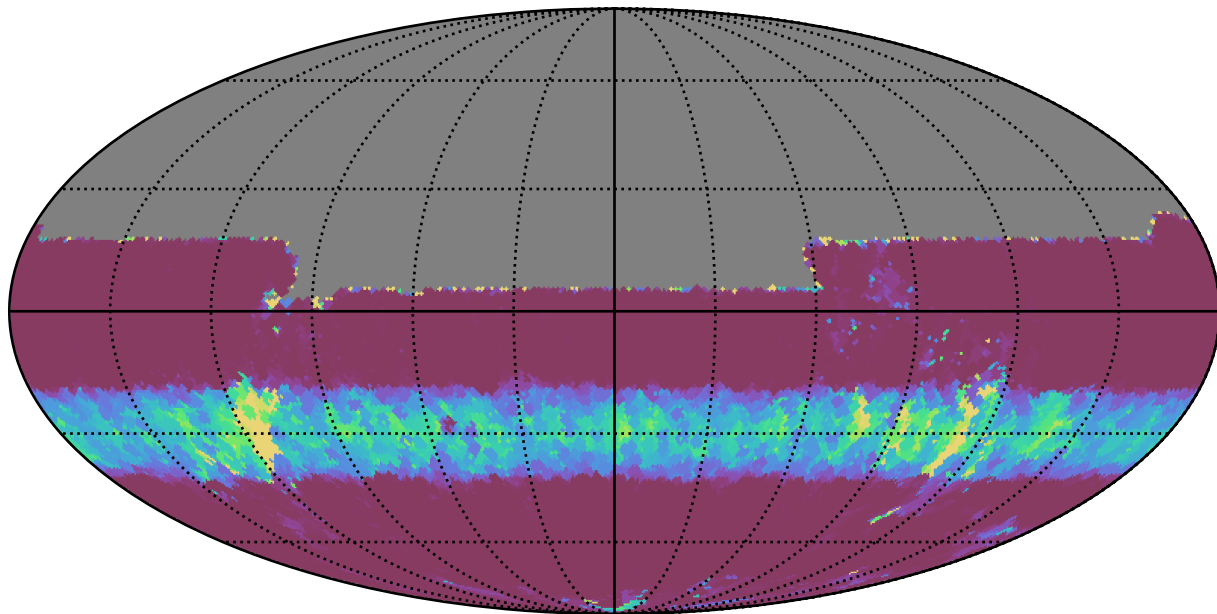
extra_ss_neo4_v3.4_10yrs All sky u band: Min normairmass
