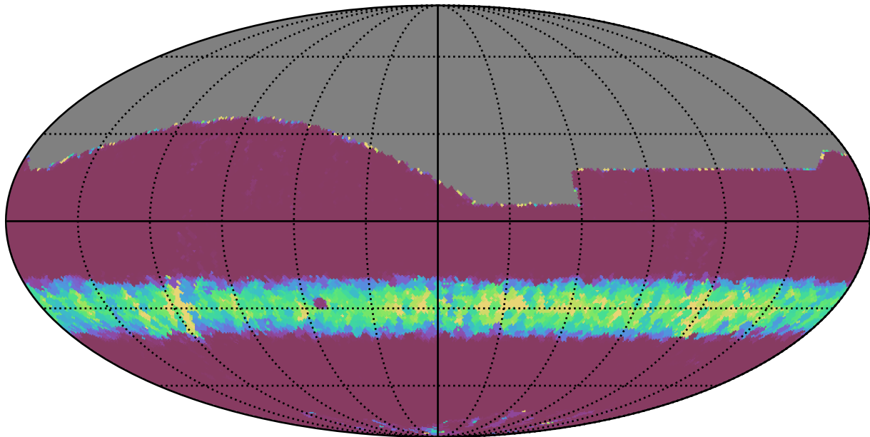
extra_ss_neo4_v3.4_10yrs All sky r band: Min normairmass
