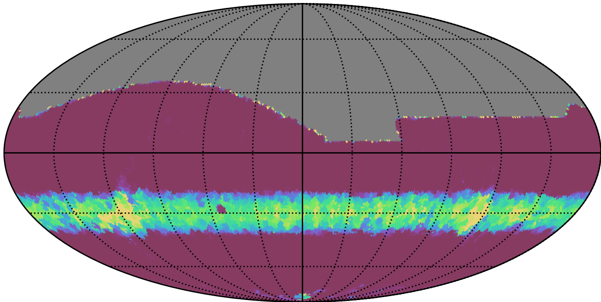
extra_ss_neo4_v3.4_10yrs All sky i band: Min normairmass
