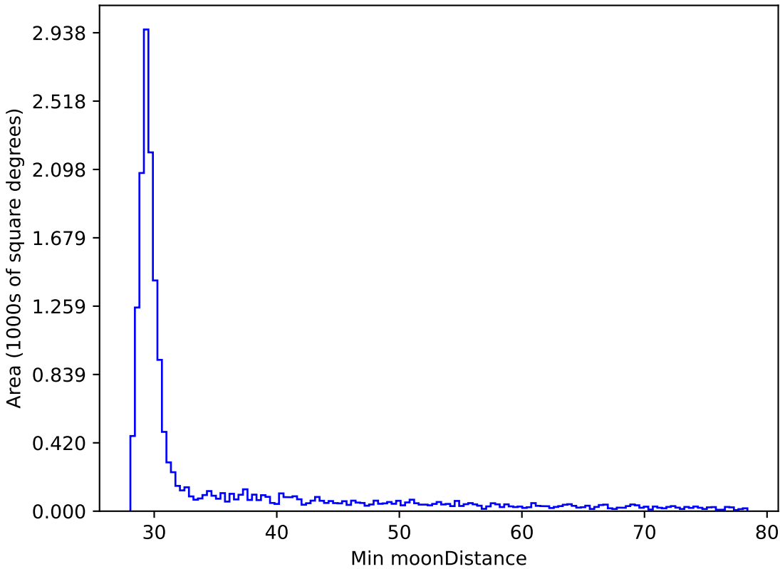
extra_ss_neo4_v3.4_10yrs WFD y band: Min moonDistance
