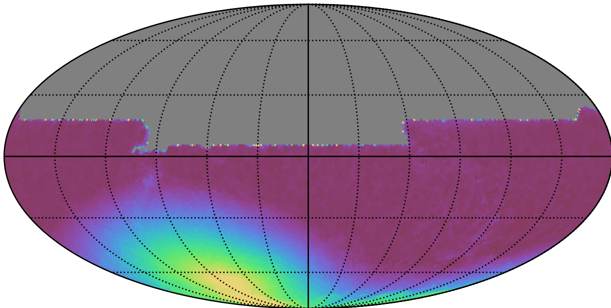
extra_ss_neo4_v3.4_10yrs All sky y band: Min moonDistance
