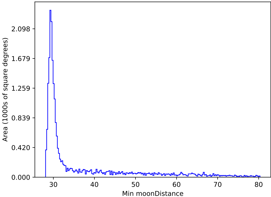
extra_ss_neo4_v3.4_10yrs All sky y band: Min moonDistance
