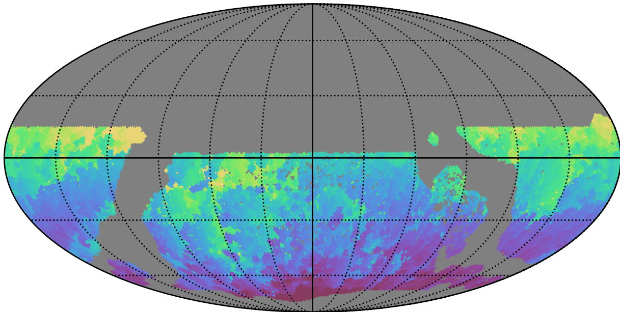
extra_ss_neo4_v3.4_10yrs WFD z band: Min HA
