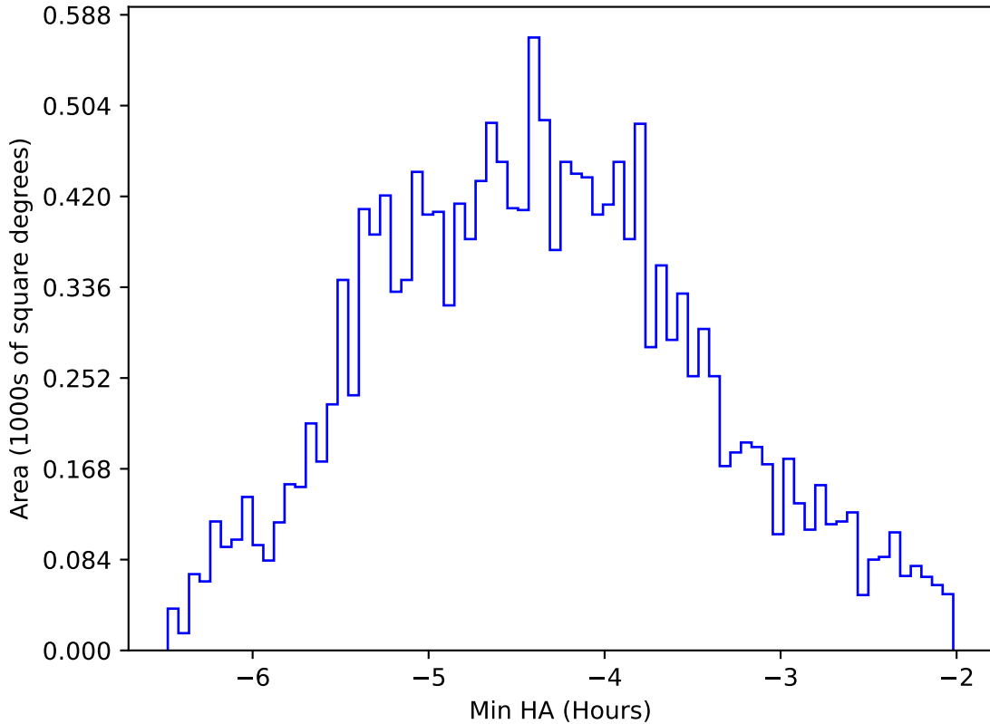
extra_ss_neo4_v3.4_10yrs WFD z band: Min HA
