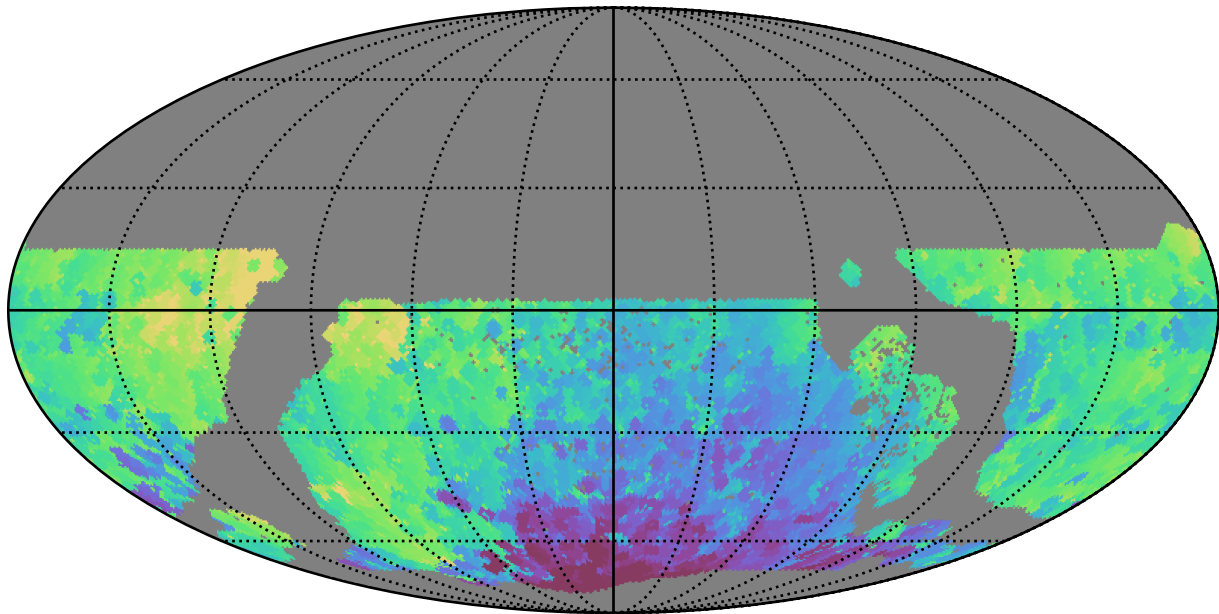
extra_ss_neo4_v3.4_10yrs WFD y band: Min HA
