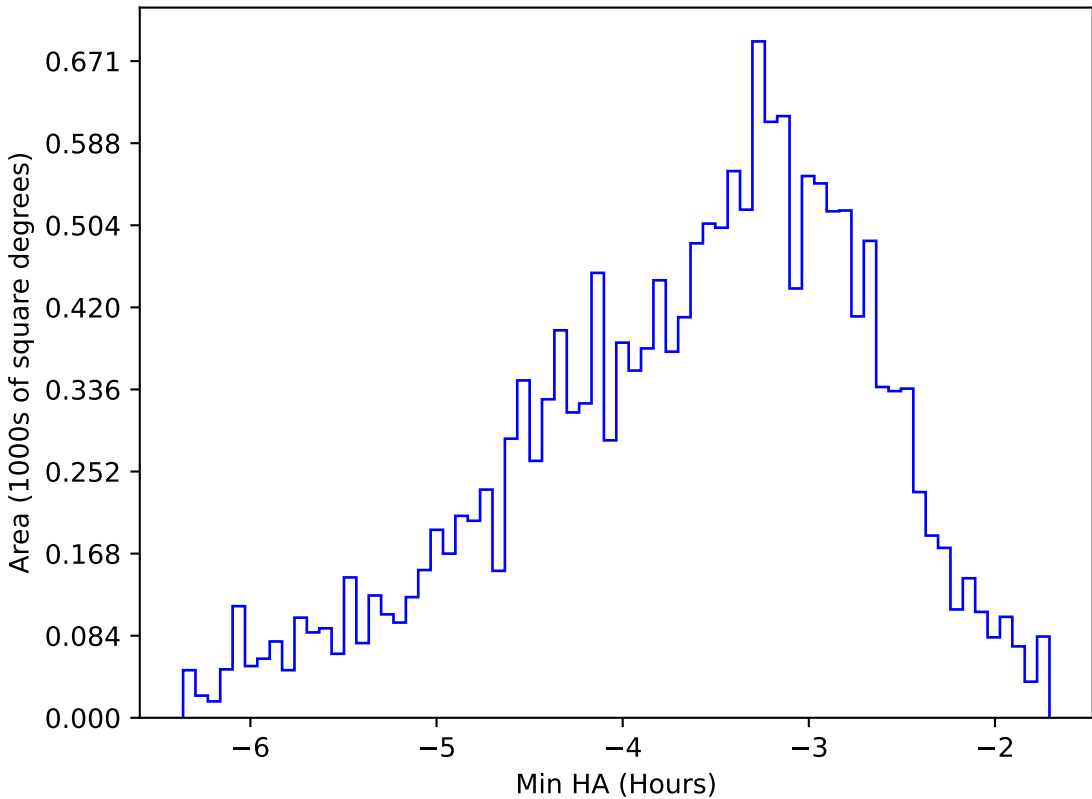
extra_ss_neo4_v3.4_10yrs WFD y band: Min HA
