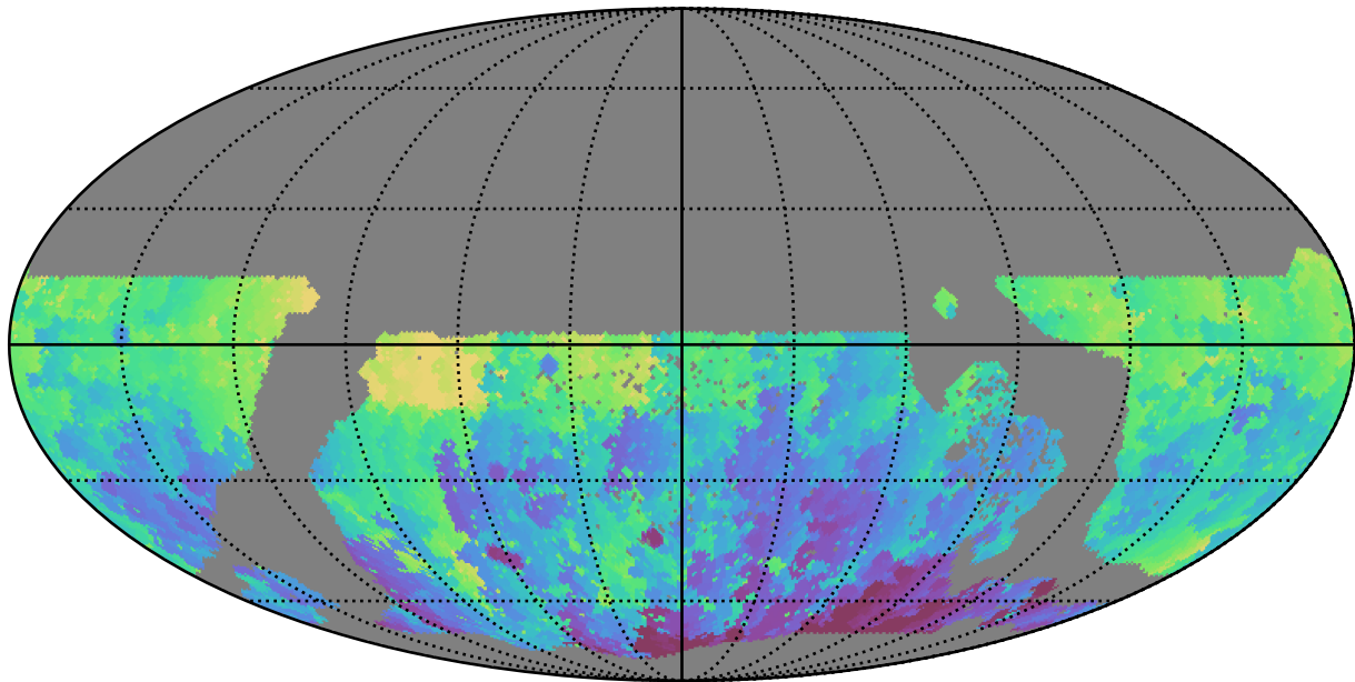
extra_ss_neo4_v3.4_10yrs WFD u band: Min HA
