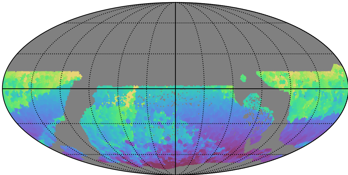
extra_ss_neo4_v3.4_10yrs WFD r band: Min HA
