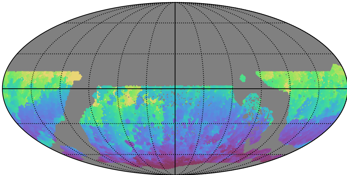
extra_ss_neo4_v3.4_10yrs WFD i band: Min HA
