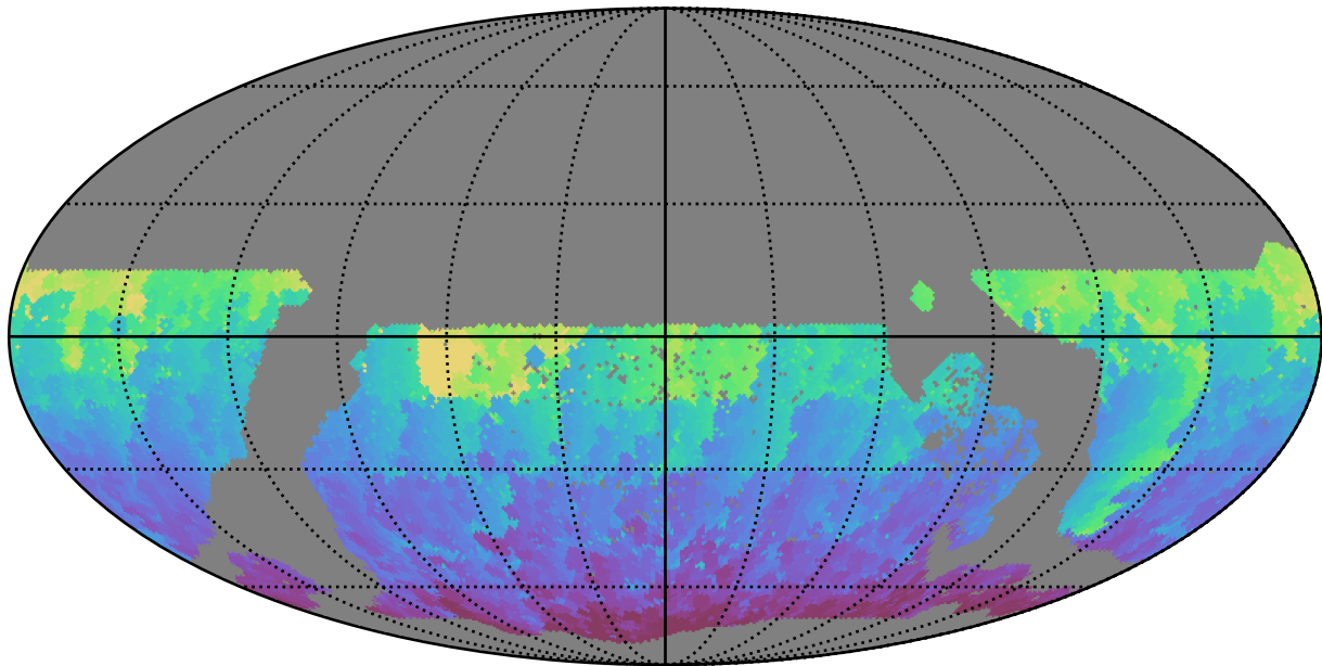
extra_ss_neo4_v3.4_10yrs WFD g band: Min HA
